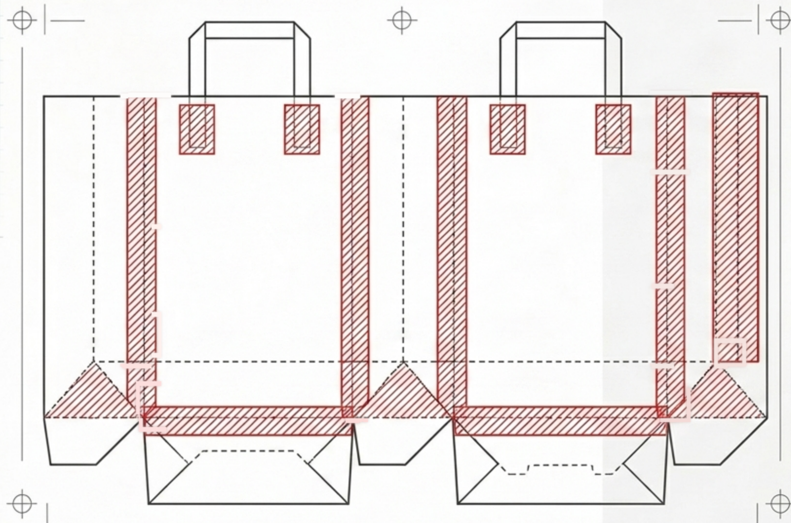
Схема развернутой высечки
